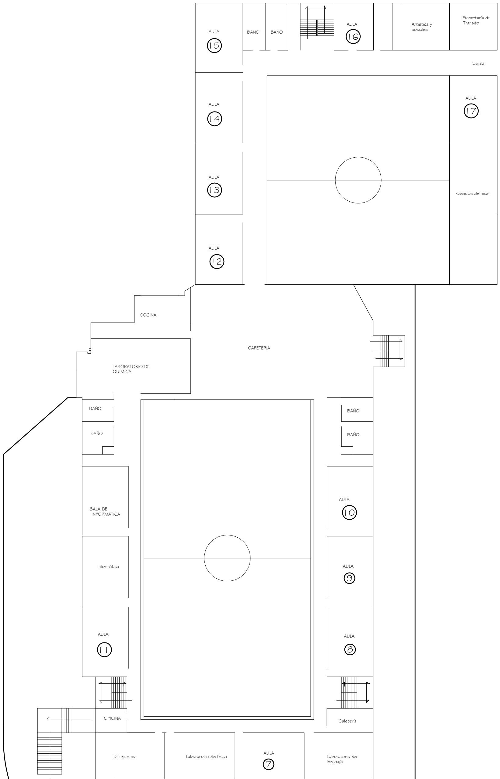
PASCUAL DE ANDAGOYA PLANTA ARQUITECTÓNICA 2º PISO ESC: 1 _____ 1
